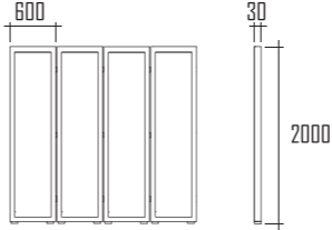
CODE : PT060000 SIZE : L600×W30×H2000mm*4
