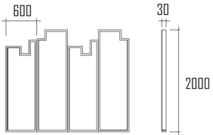
CODE : PT070003 SIZE : L600×W30×H2000mm*4
